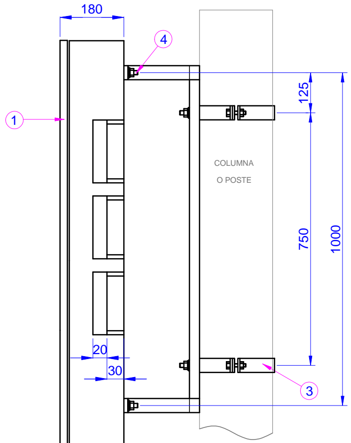
VISTA LATERAL MONTAJE s/ Esc.
