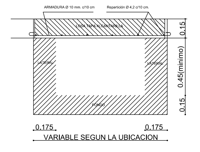
LOSA TAPA: Hormigón simple de 350 kg de cemento por m³ H-21 FONDO Y LATERALES: Hormigón simple de 250 kg de cemento por m³ H-13 FIERRO: fy = 400 kg/cm²
