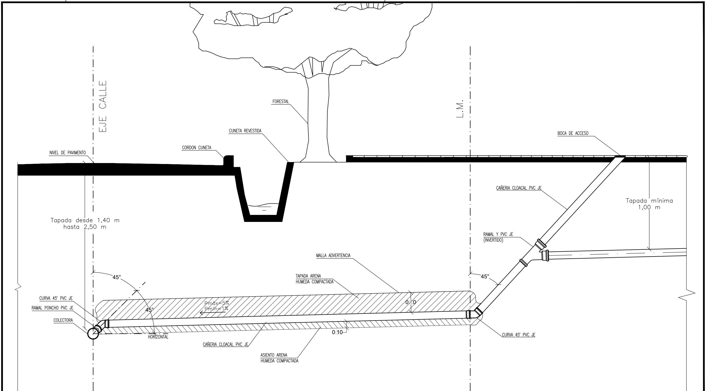
CORTE ESQUEMATICO
