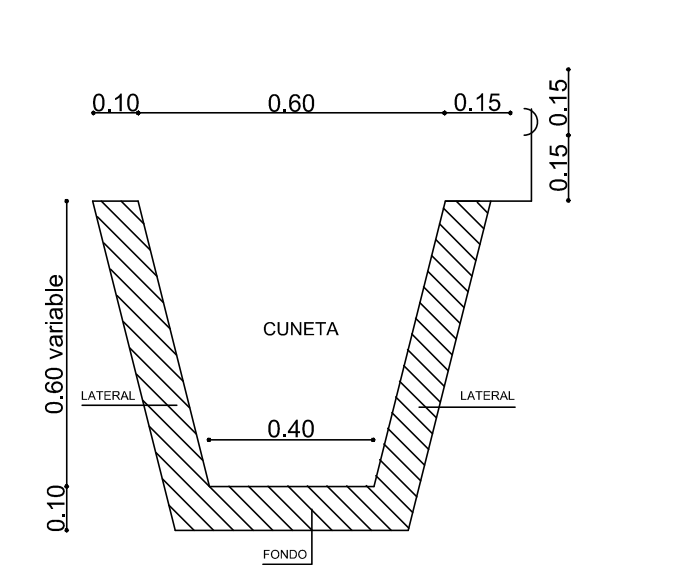
CORDON: Hormigón simple 350 kg de cemento por m³ H-21 FONDO Y LATERALES: Hormigón simple 250 kg de cemento por m³ H-13
