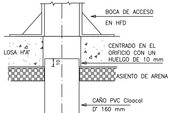
DETALLE HUELGO
