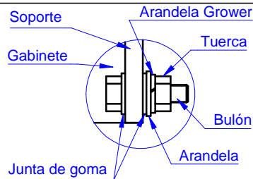
DETALLE A Fijación Gabinete-Soporte
