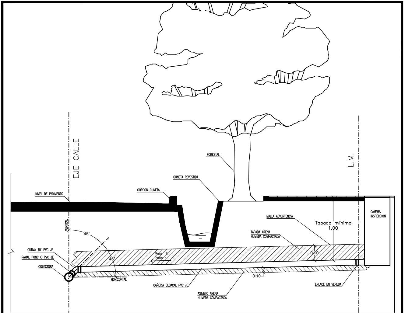
CORTE A-A
