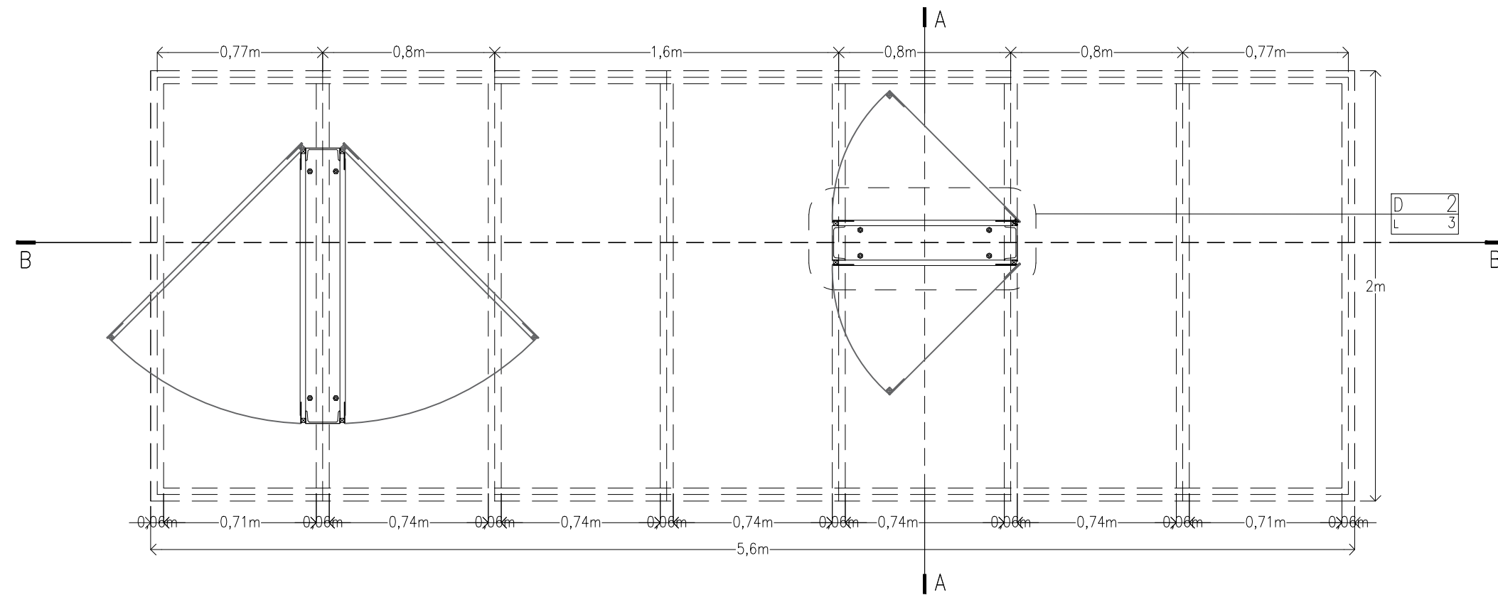
PLANTA +1.4 M
