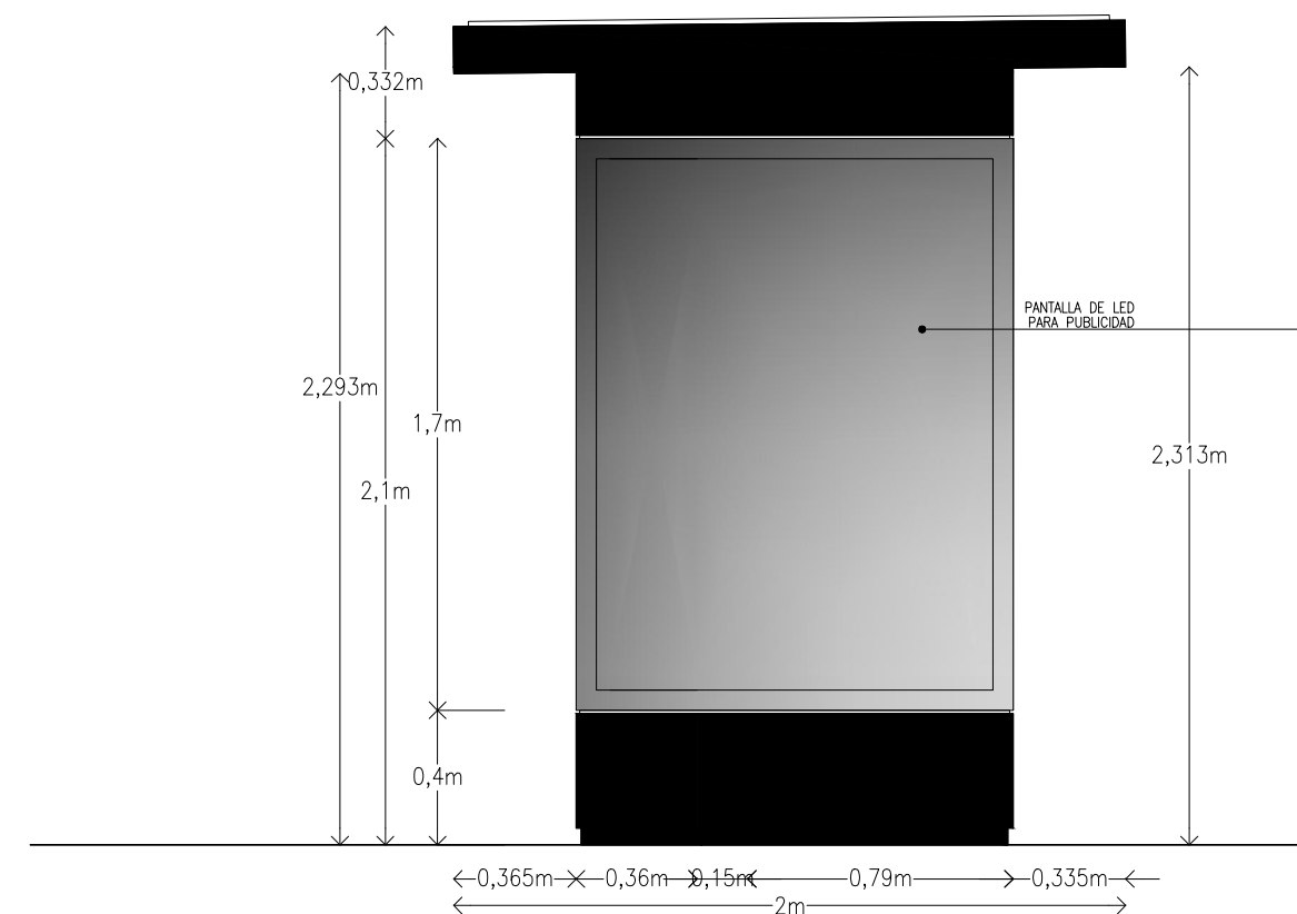
VISTA LATERAL
