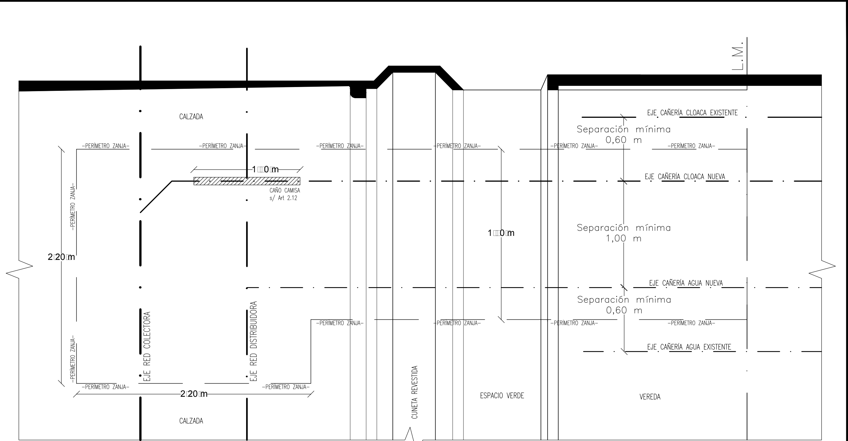
PLANTA
