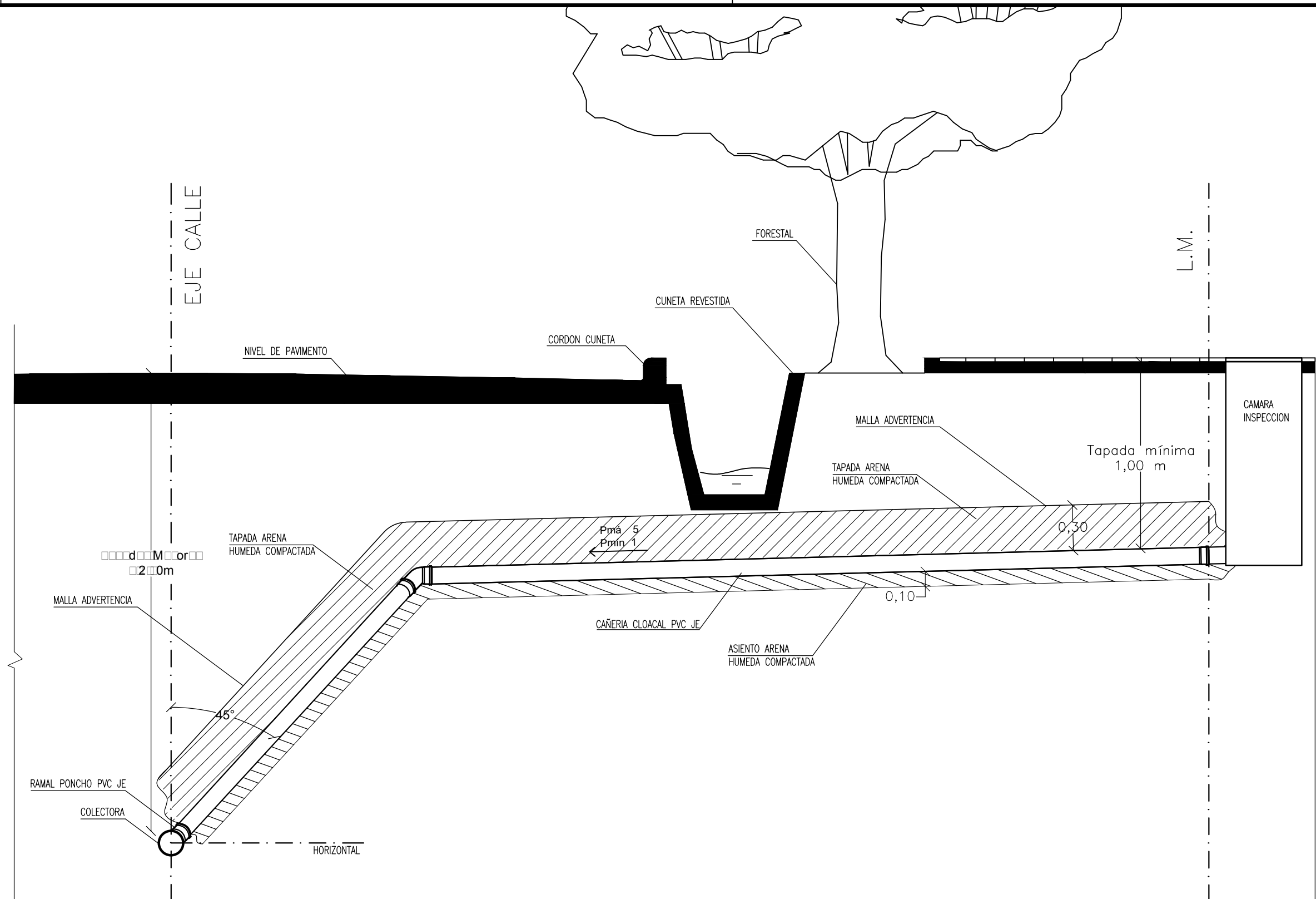
CORTE ESQUEMATICO
