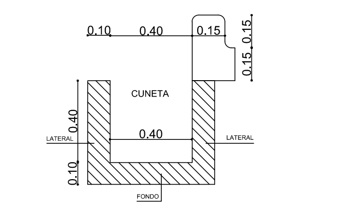
CORDON: Hormigón simple 350 kg de cemento por m³ H-21 FONDO Y LATERALES: Hormigón simple 250 kg de cemento por m³ H-13
