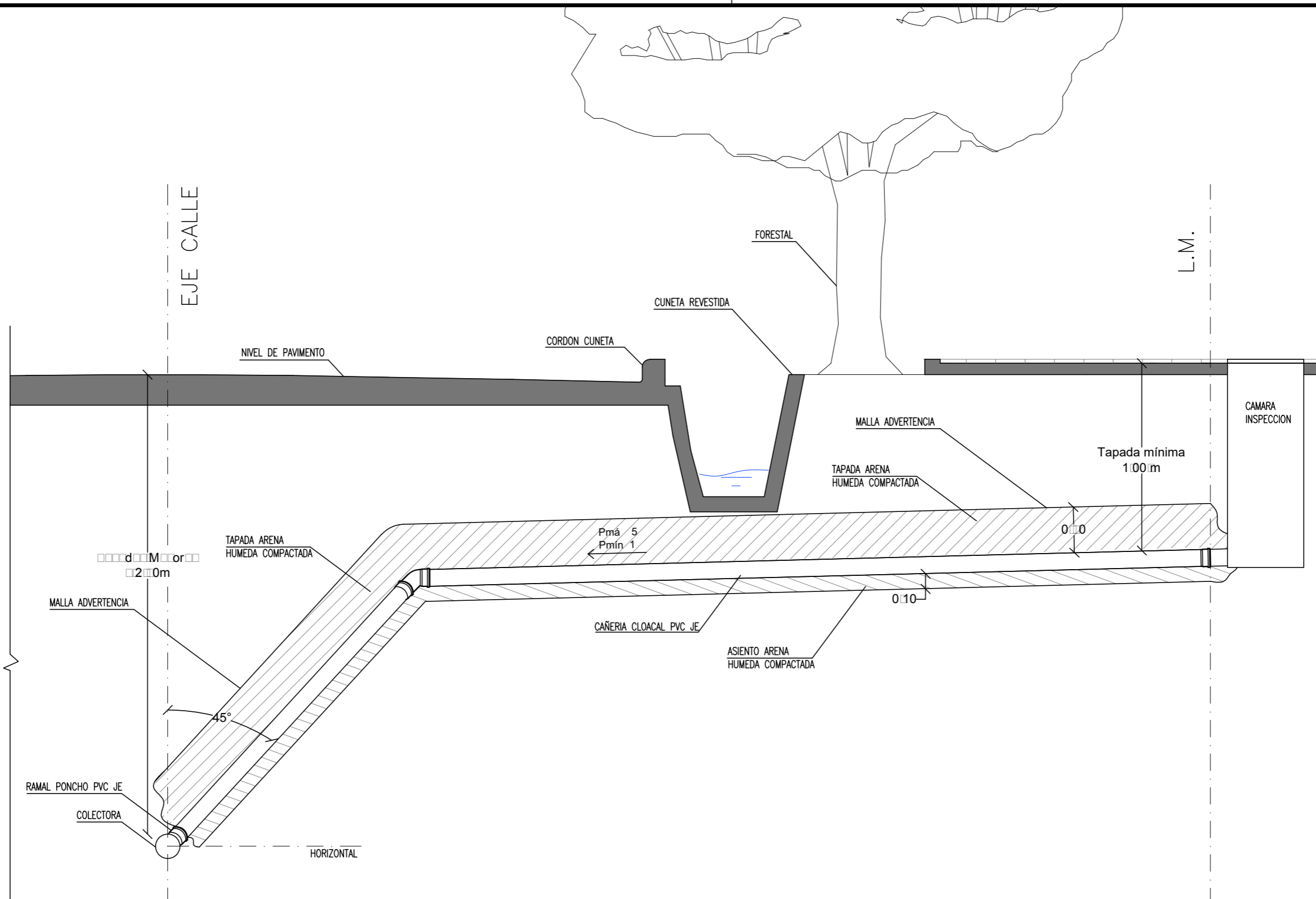
CORTE ESQUEMATICO
