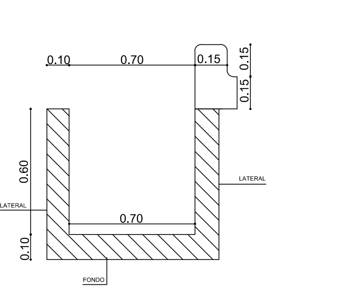
CORDON: Hormigón simple 350 kg de cemento por m³ H-21 FONDO Y LATERALES: Hormigón simple 250 kg de cemento por m³ H-13
