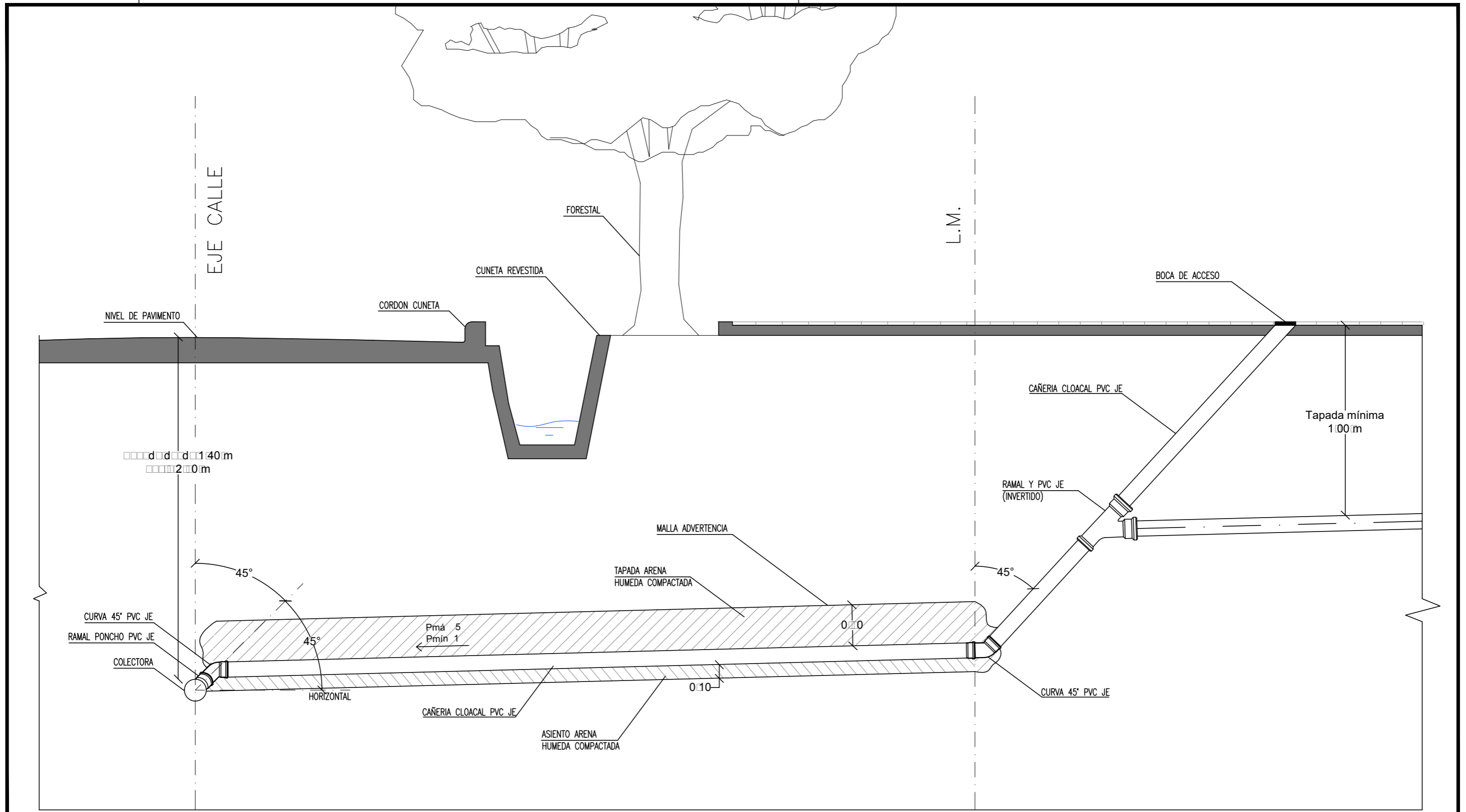
CORTE ESQUEMATICO
