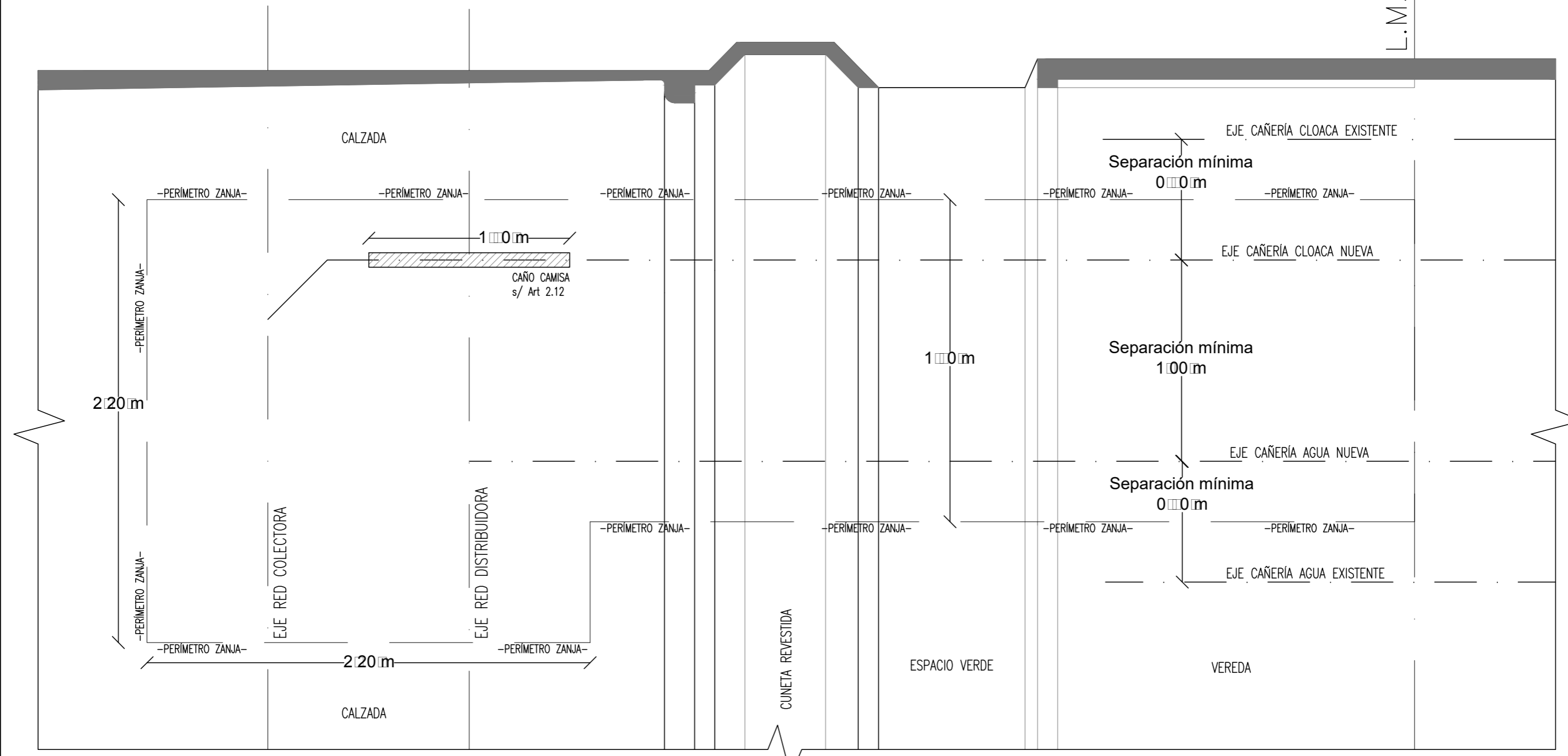
PLANTA
