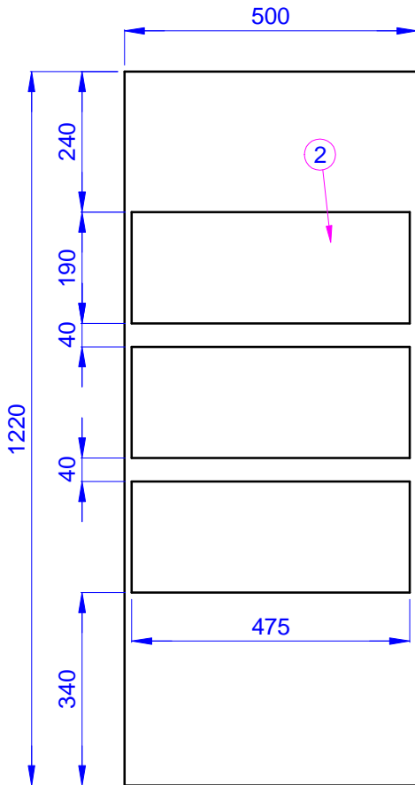
VISTA FRENTE MONTAJE s/ Esc.
